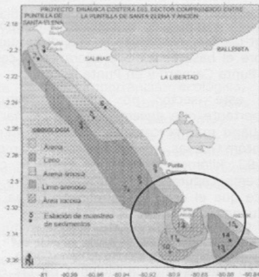
Figura 8.- Mapa de distribución aproximada de los sedimentos según su textura.
