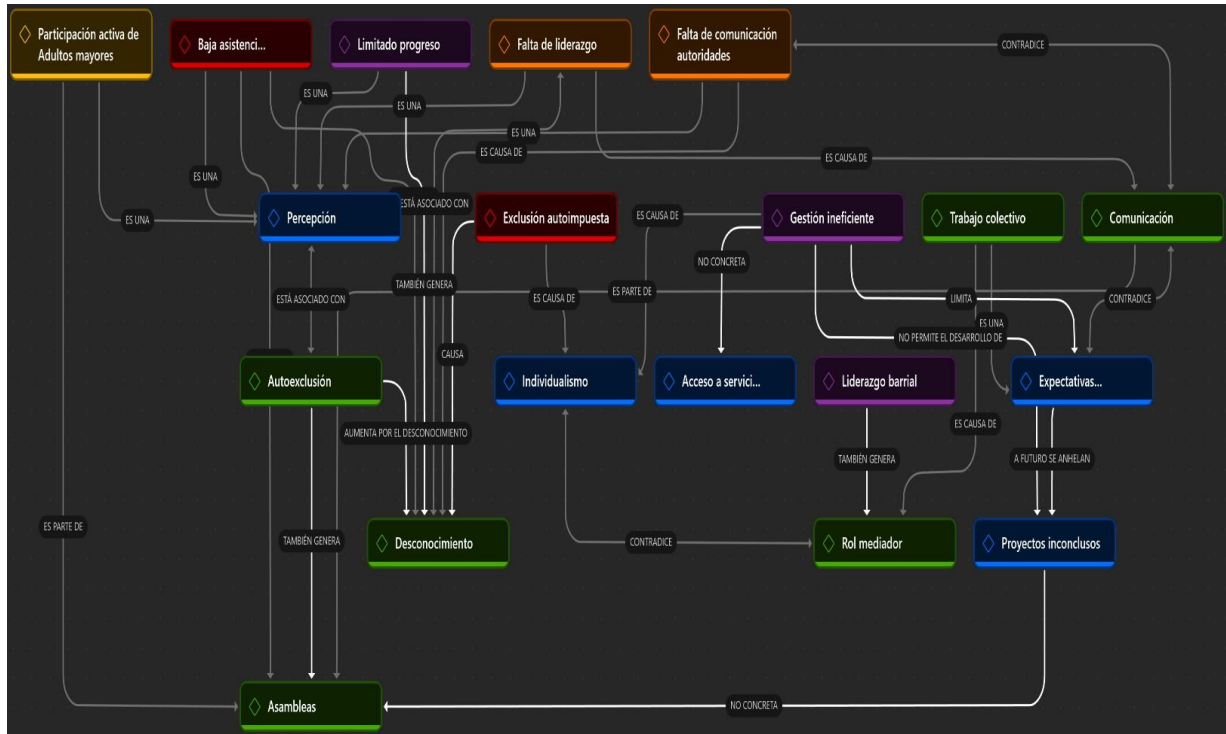
Figura 1 Red semántica
