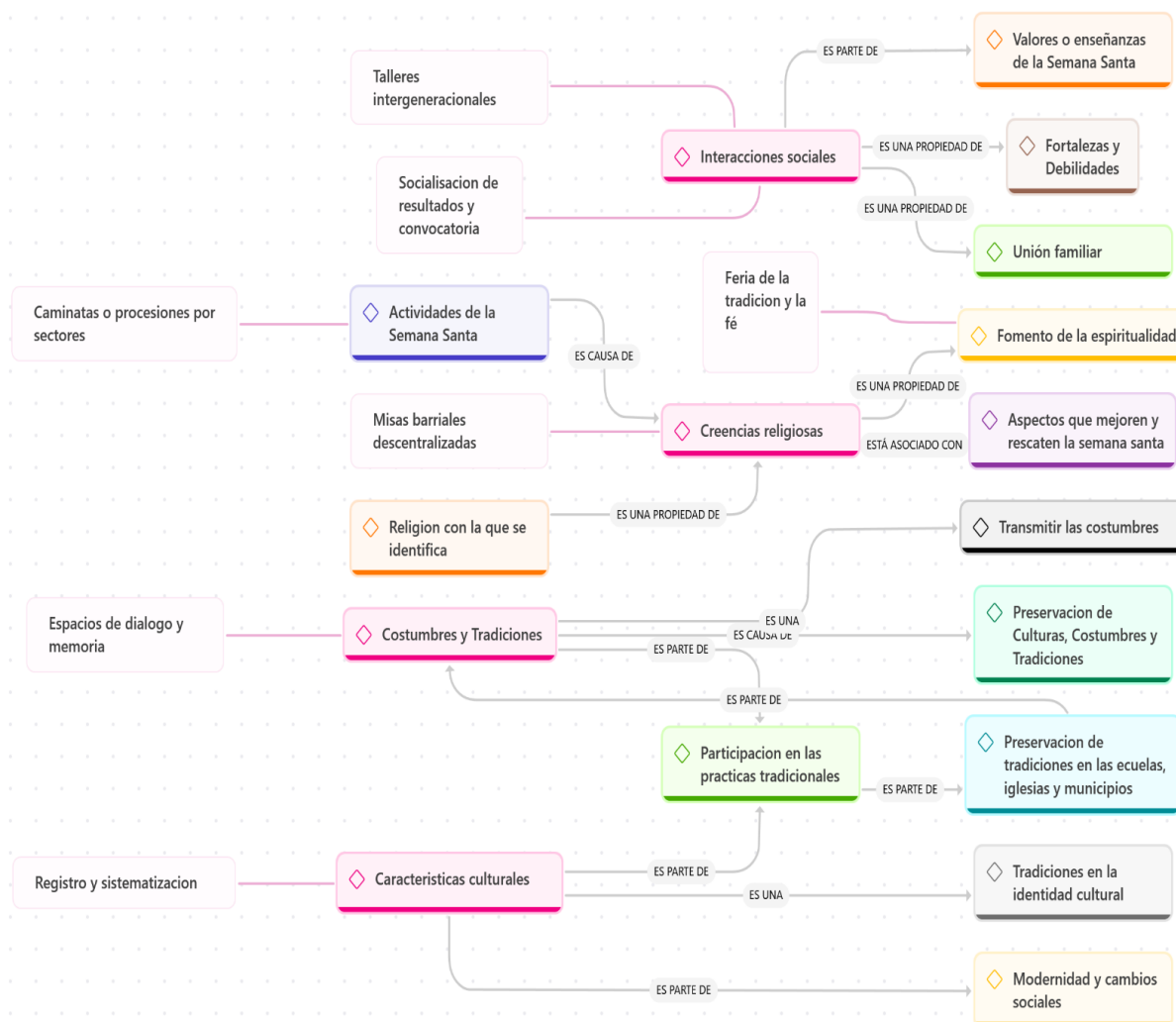
Figura 1 Red semántica
