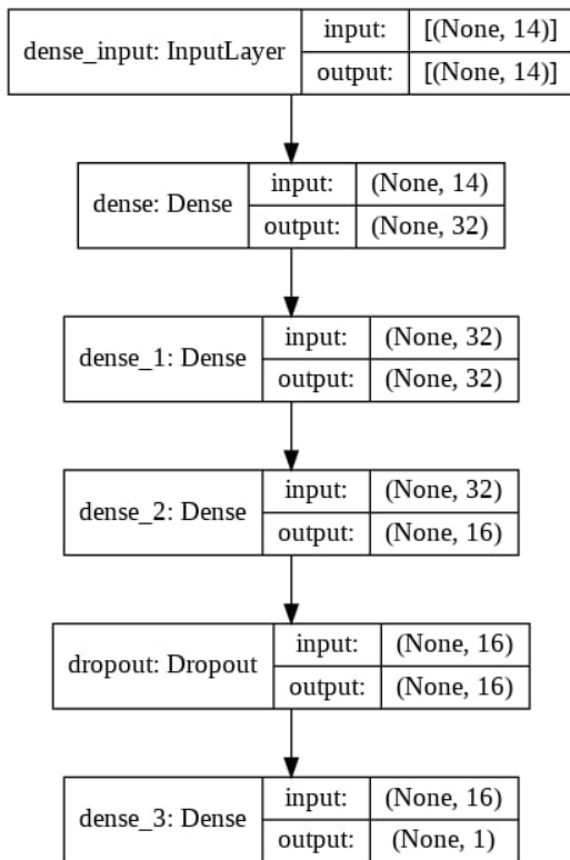
Figura 5. Arquitectura de la red neuronal.
