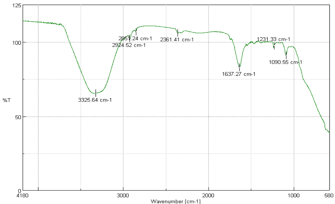
Figura 4. Identificación de grupos funcionales por Espectroscopía Infrarroja para Chlorella vulgaris . Fuente: Autoría propia
