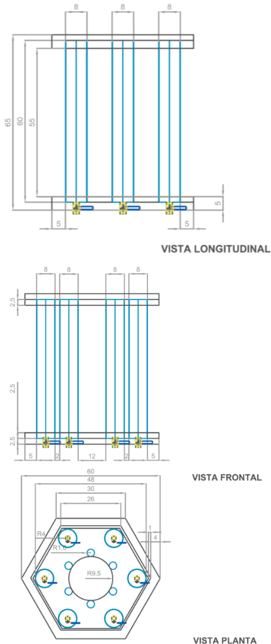
Figura 1. Fotobiorreactor discontinuo. Fuente: Autoría propia
