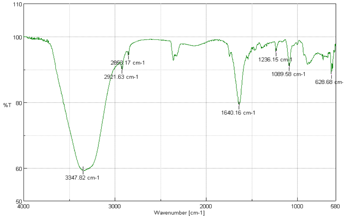
Figura 5. Identificación de grupos funcionales por Espectroscopía Infrarroja para Scenedesmus . Fuente: Autoría propia
