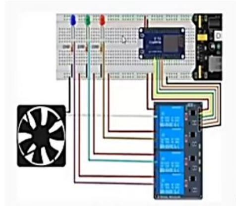
Figura 2: Diseño y simulación del proyecto.
