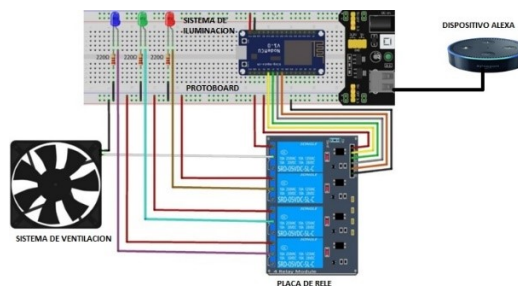
Figura 4: Diseño eléctrico.
