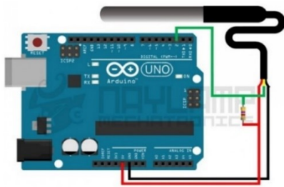
Figura 4: Sensor de temperatura DS18B20. Fuente: [15]
