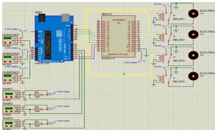
Figura 10: Diseño electrónico del sistema de riego inteligente
